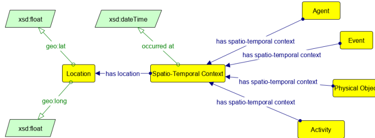
Fig. 2. Spatio-Temporal Context
